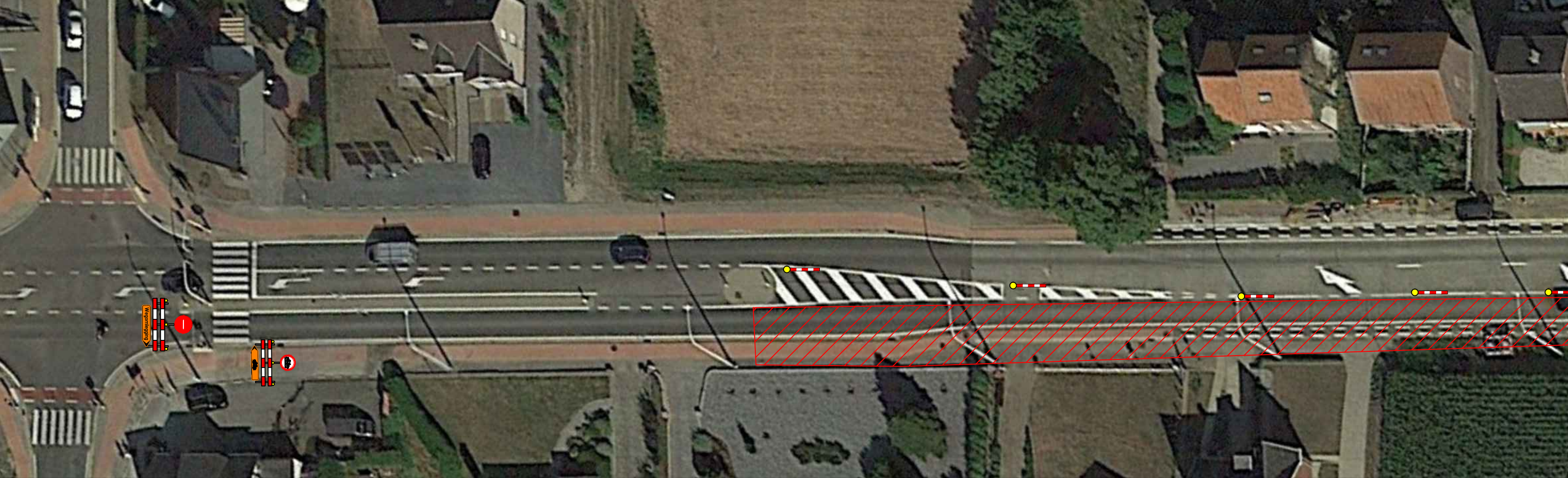
Detail kruispunt Schillekensberg
