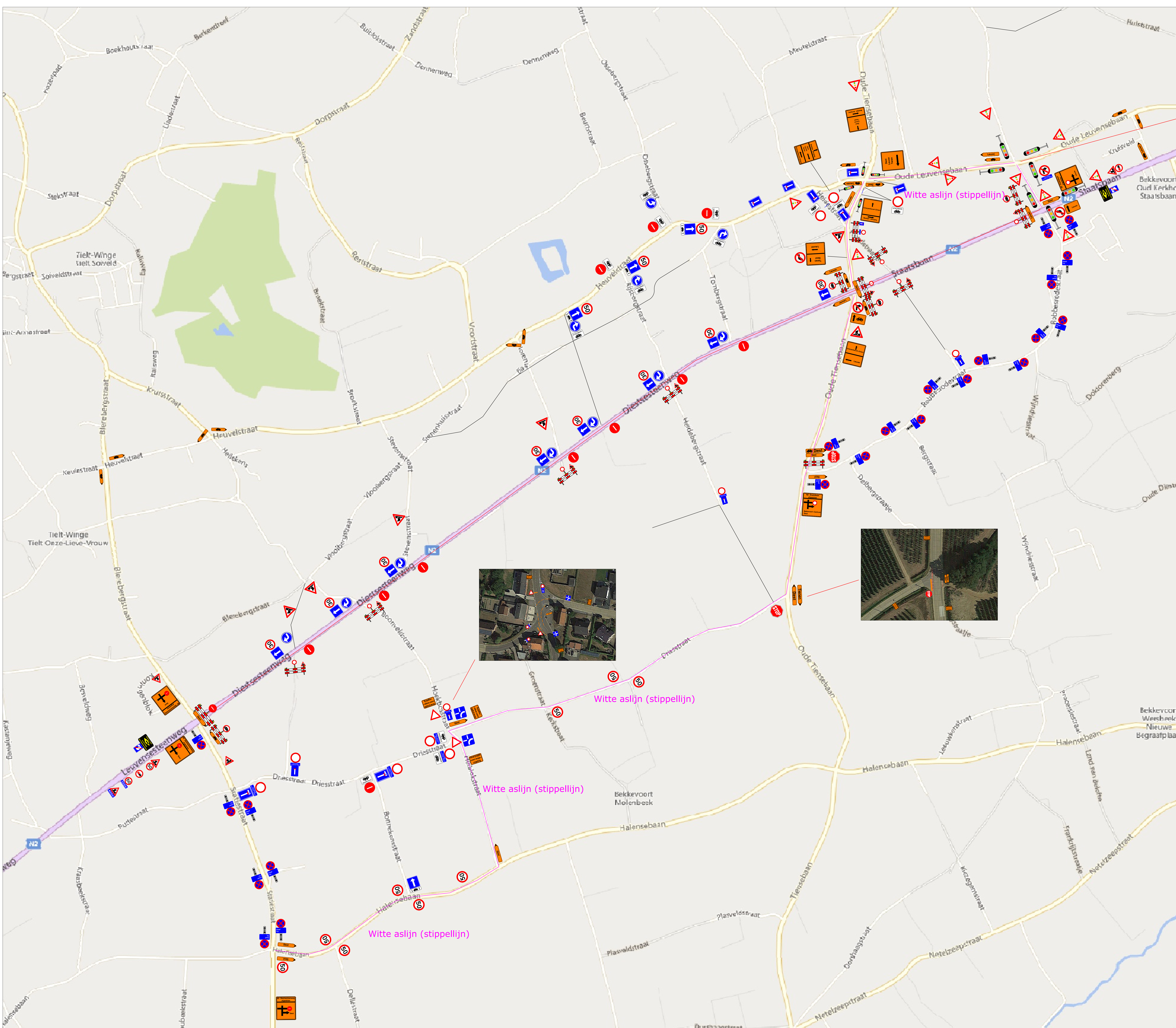
Detail kruispunt Oude Tiensebaan
